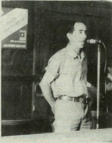
Moises Jaso Gaintzakoa orain dela hogeit bat urte plazaz plaza bertsolari onenekin ibilia.
