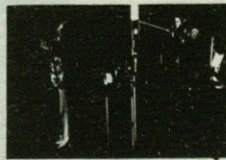
Urteetan aritu da Herri Irratian, Populandia, El jazz y otras músicas, eta musika-programak egiten, beste irrati-gizon asko ez bezala honestitate, dignitate, eta kalitate minimo batekin.
