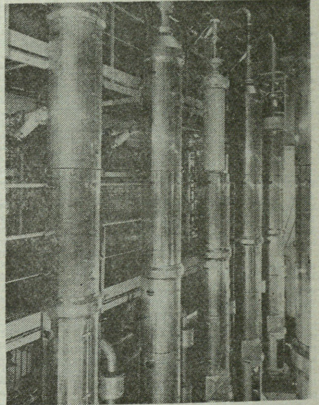
Frantziako «Eurodif» lantegian uranioa aberasteko erabiltzen diren «difusioerak».
