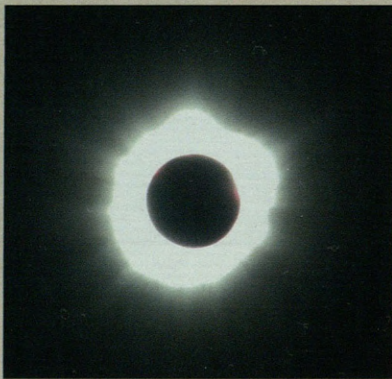
Eguzki eklipsea.
