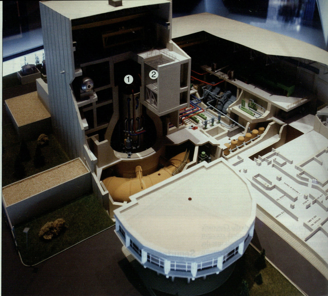
Garoiako zentrala barrutik irudikatzen duen maketa. Agertzen diren eraikinetara debekatuta dago sarrera. Besteak beste erreaktorea (1) eta erradioaktibitate altuko hondakinen igerilekua (2) ikus ditzakegu. Uranioa igerilekuaren hondoan kokatzen da.
