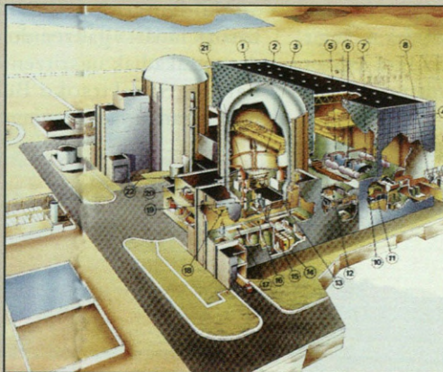
Zentral nuklearren funtzionamendua azaltzeko eskema.
