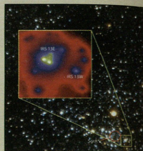
IRS 13 deituriko eremu distiratsua aztertu dute, batez ere, bertan biraka ari den izar-taldea.
