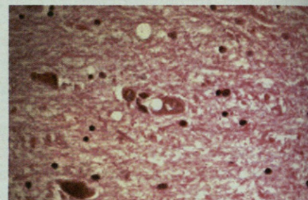
■ Entzefalopatia Espongiformea gaitza gizakiaren garunean.
