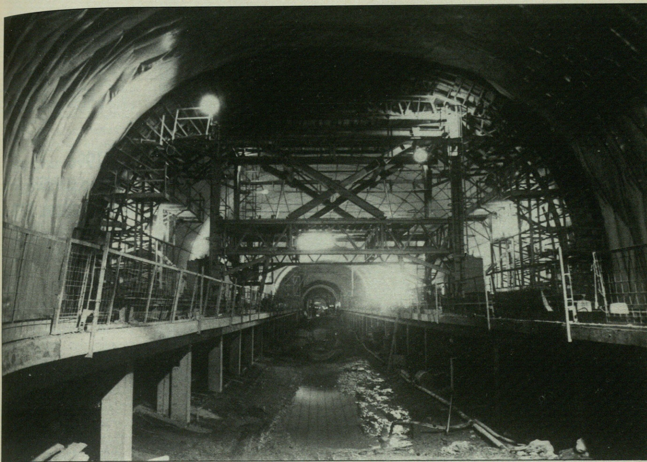
41 kilometroko luzerako tunel hauek makina marruskagarrien bidez egin dira; egunero hiru metroko zuloa egiteko ahalmena dute.
