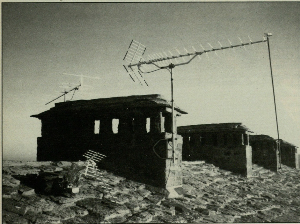
Hona hemen Paz de Zigandak ikastolak Aralarreko San Migelen jarritako errepikagailua.
