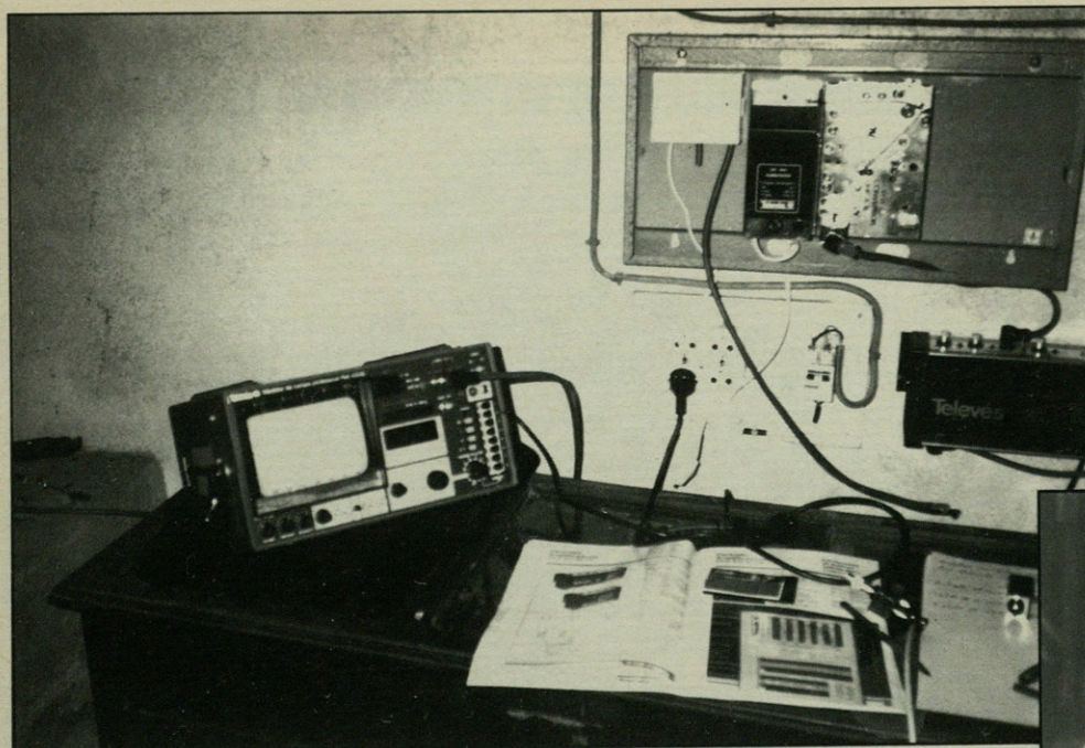
San Migeleko errepikagailuaren hasieran erabilitako aparailu osagarriak. Behean, Rafa Zazpe montaia guztiaaren tekniko.
