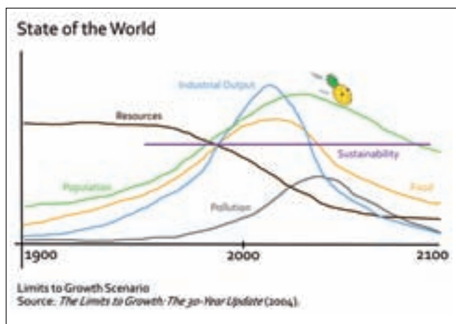
“Limits to Growth”-en 2004ko argitalpeneko grafiko famatua. Kurbek irudikatzen dituzte: Baliabideak, Industriaren emaitzak, Kutsadura, Populazioa eta Janaria.
